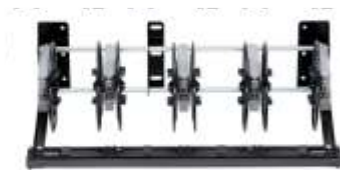
Nella superficie possono essere installati fino a 5 porta bobine avitabili nei fori predisposti con viti M5.
